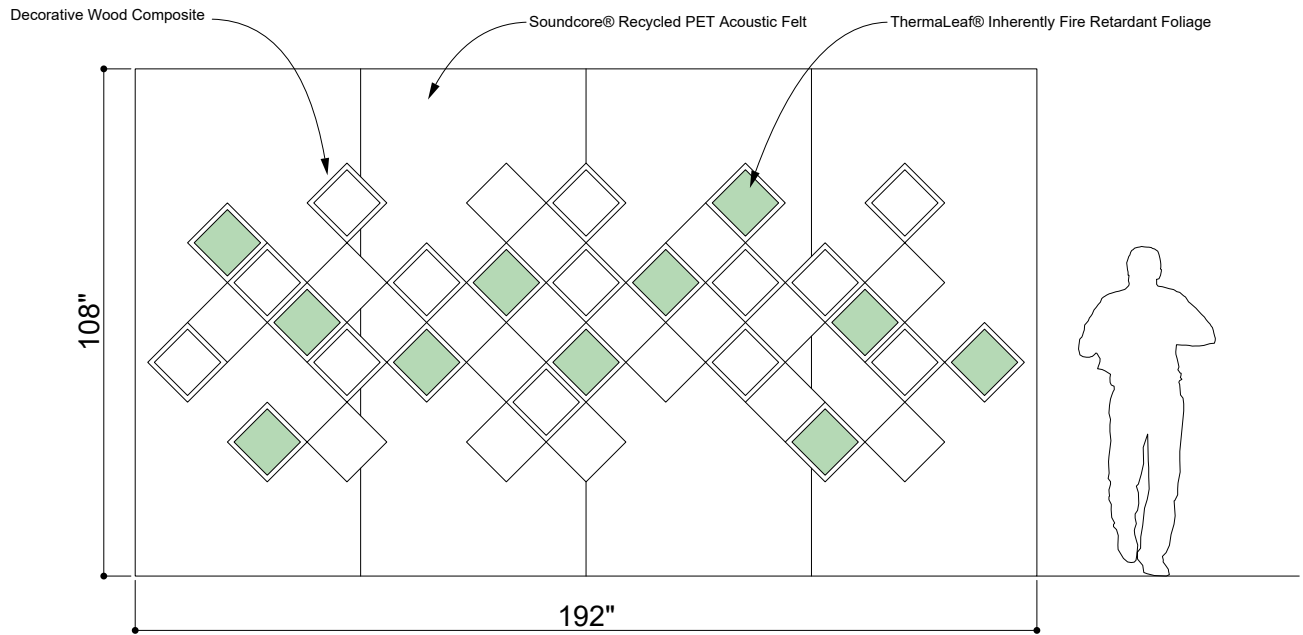
① ELEVATION 1
